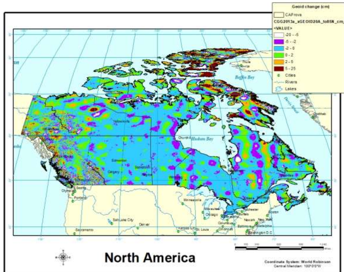
CGG2013a – xGEOID20A
